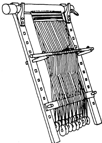
Tyngdvävstol med stomme av två stöttor som lutar mot vägg e.d. Varpen sträcks med tyngder.
